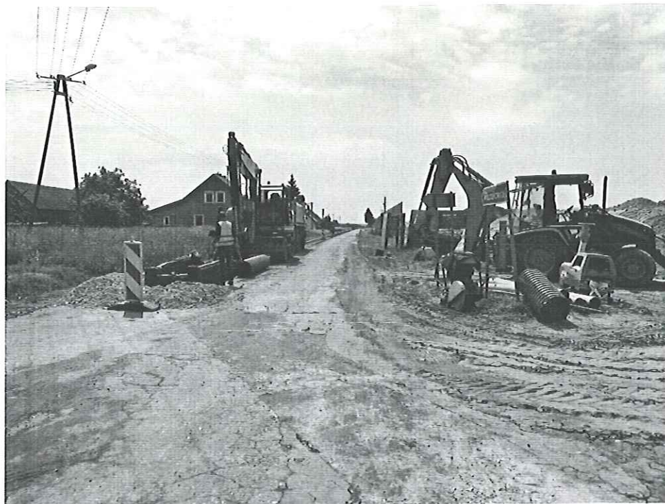
Dalszy etap budowy kanalizacji w Dłużynie
