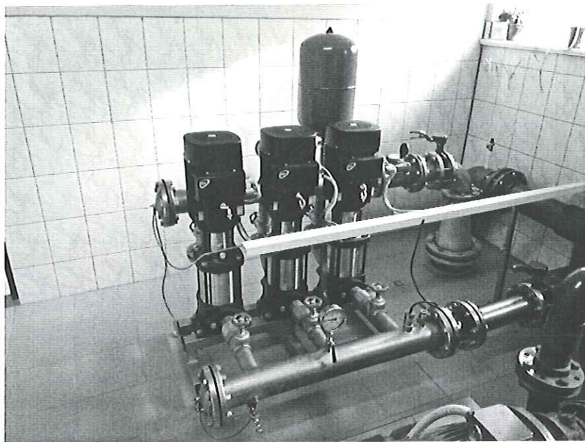
Nowy odrębny zestaw sieciowy na SUW Włoszakowice
